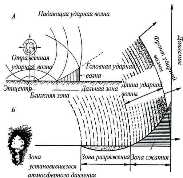
Рисунок 7 – Формирования ударной волны при воздушном ядерном взрыве. А – отраженная ударная волна накладывается на падающую ударную волну и нагнывает с тыльной стороны на зону сжатия падающей волны, сливаясь с ней – образует головную ударную волну большего давления. Б – структура ударной волны [19]
